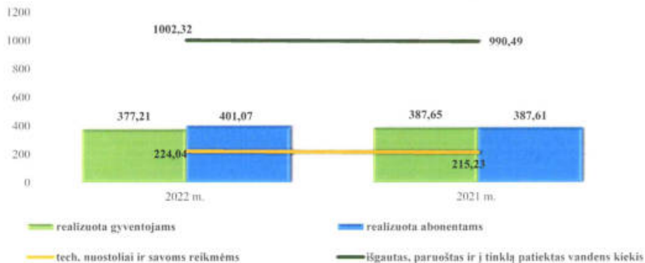
12 paveikslas. 2021 m. ir 2022 m. išgauti, paruošti, į tinklą patiekti ir realizuoti geriamojo vandens kiekiai, tūkst. m 3
